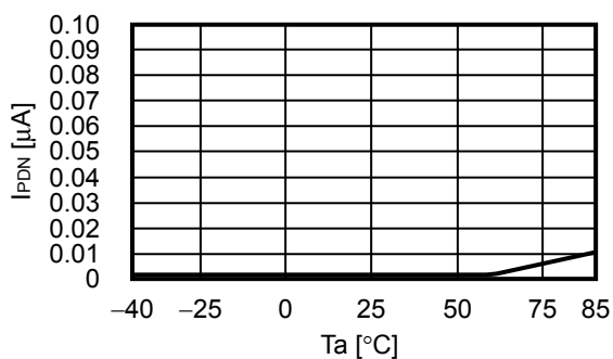
1.4 I_{PDN} - T_a
