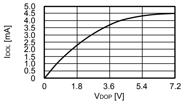
4.4 I_{DOL} - V_{DOP}
