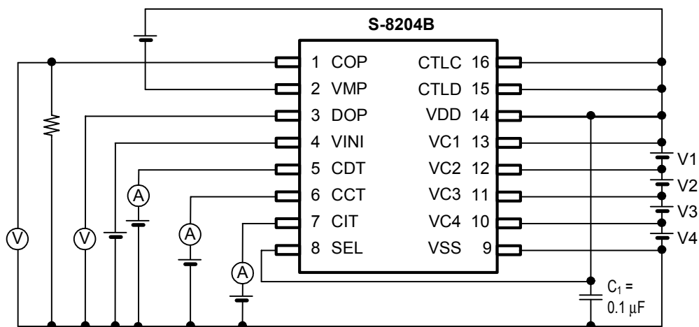
图6 测定电路3
